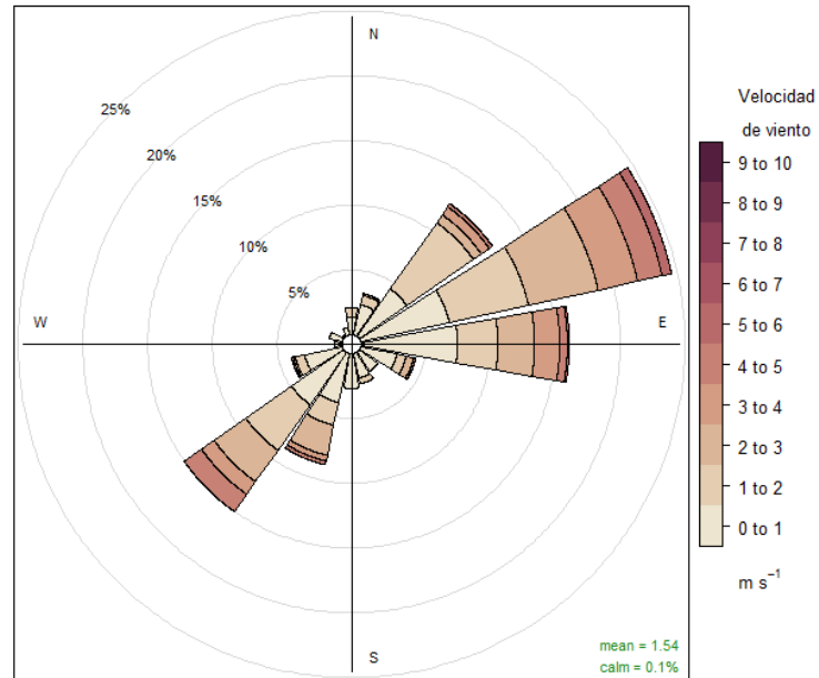
Frecuencia por dirección de viento (%)
