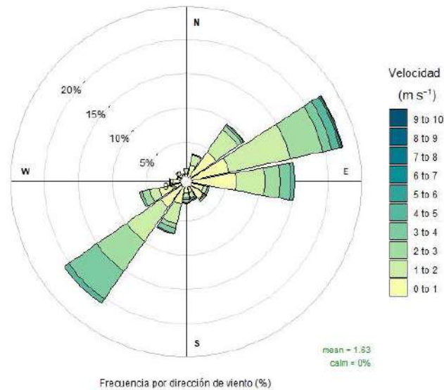
Gráfica 7. Rosa de Vientos ZMQ, mayo 2026.
